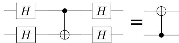
Fig. 4 Cnothadamard Basis
